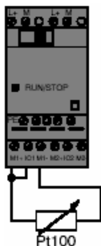
2-проводное подключение
